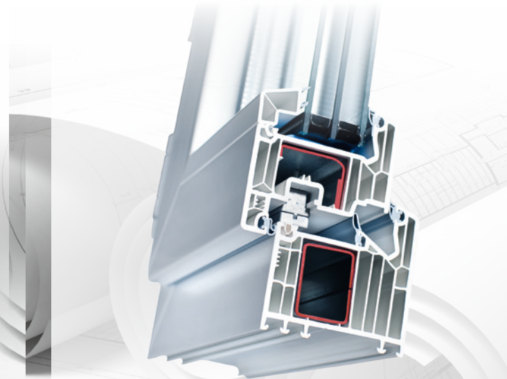
3 Profile für Rahmen, Flügel und andere Konstruktionselemente
